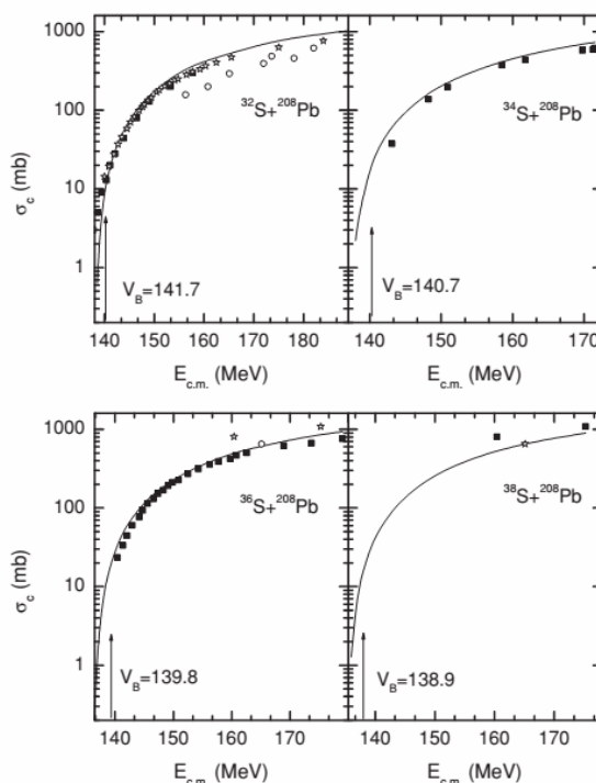
Рис. 7. Рассчитанные сечения захвата (сплошные кривые) для указанных реакций
