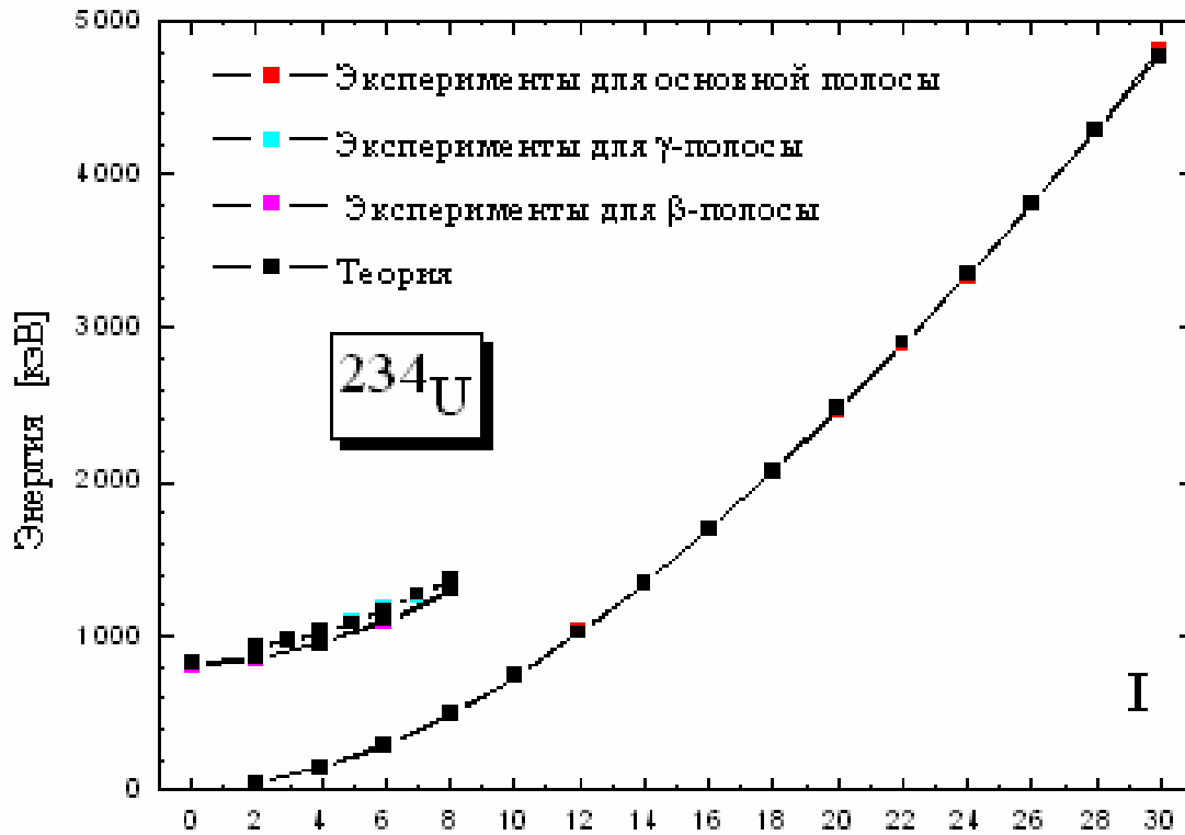
Рис. 2. То же самое как в рис. 1, но для ядра ^{234}\text{U} ( \hbar\omega=408.3 keV; \mu_\beta=0.2219 ; \mu_\gamma=1.0272 ; \gamma_0=8.3^\circ ; RMS=12.1 keV).
