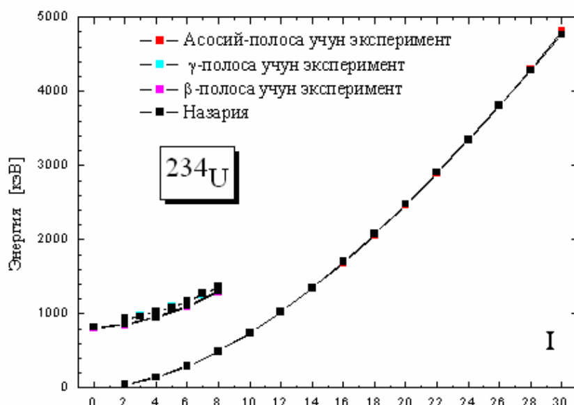
2-расм. Худди 1 расмдагидек, аммо ^{234}\text{U} ядроси учун ( \hbar\omega=408.3 keV; \mu_\beta=0.2219 ; \mu_\gamma=1.0272 ; \gamma_0=8.3^0 ; RMS=12.1 keV)
