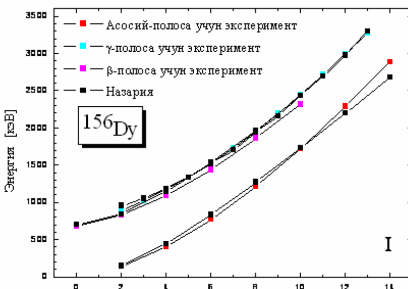
1-расм. ^{156}\text{Dy} ядросининг уйғонган ҳолатларнинг энергетик спектрининг назарий ва экспериментал қийматлари ( \hbar\omega=349.4 keV; \mu_\beta=0.4383 ; \mu_\gamma=0.893 ; \gamma_0=13.9^0 ; RMS=64.94 keV)
